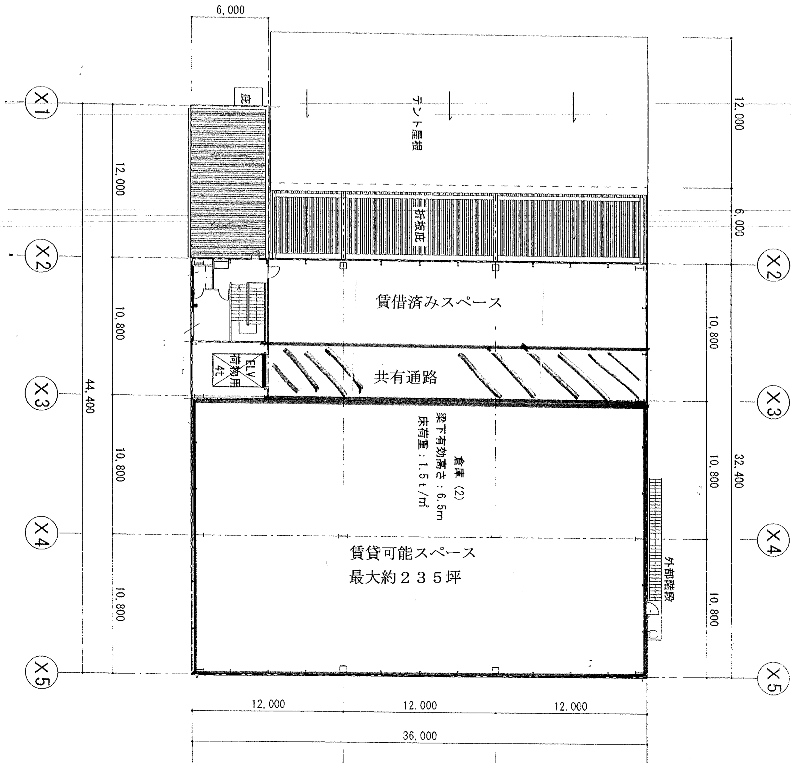
倉庫 2 F 平面図
