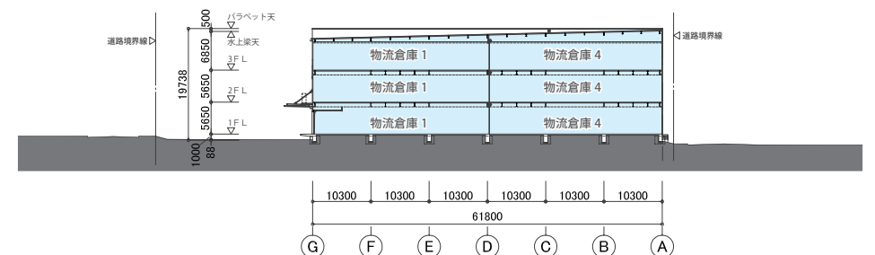
B - B 断面図 S=1/1200
