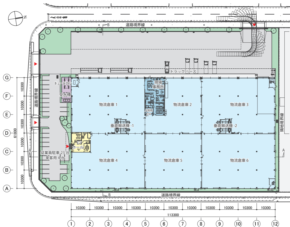
配置図兼 1 階平面図 S=1/1200
