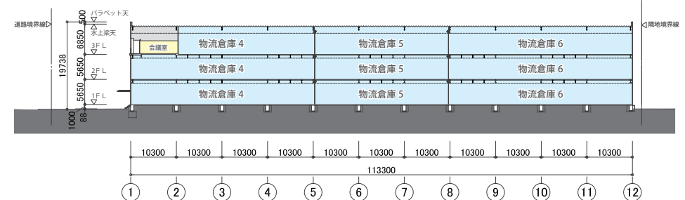
A - A 断面図 S=1/1200
