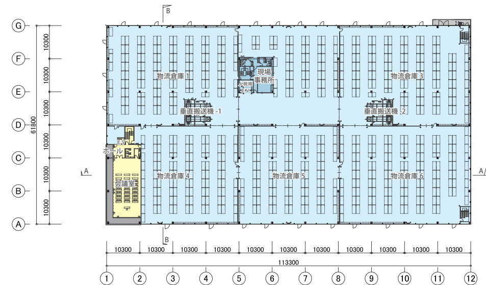
3 階平面図 S=1/1200
