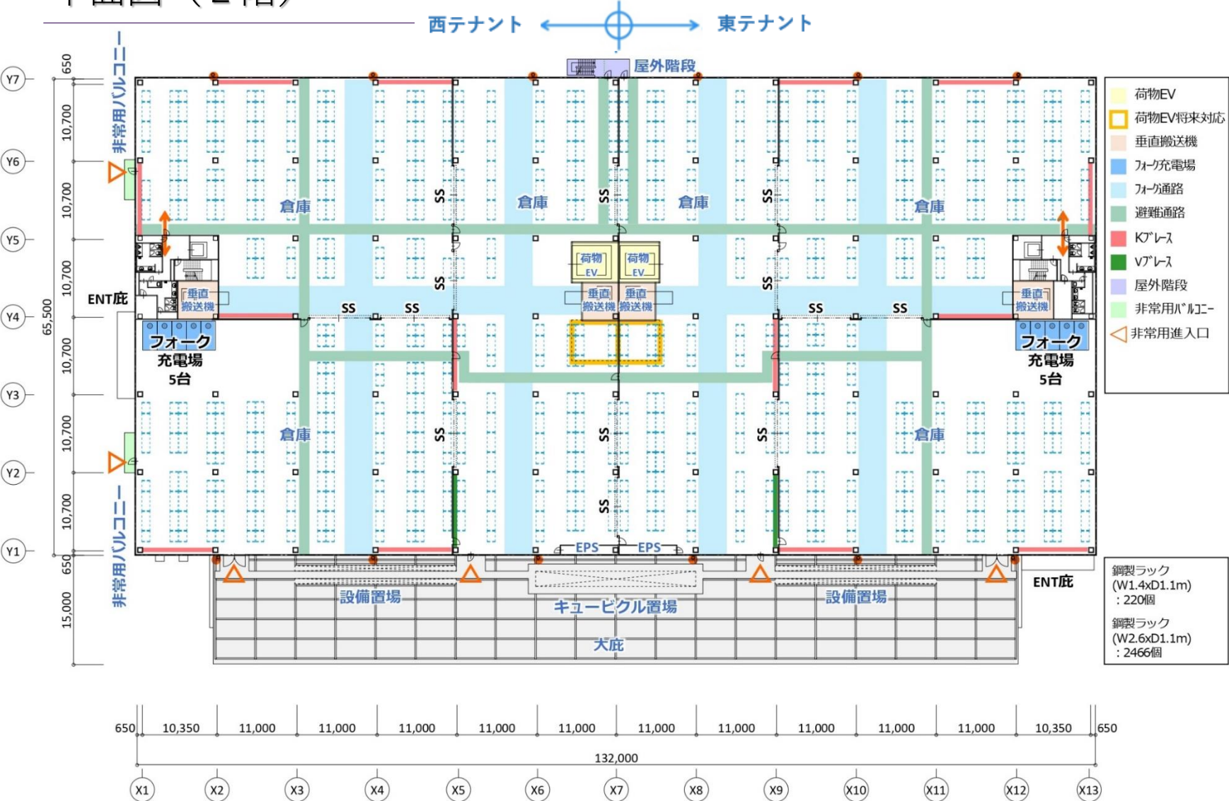
平面図（2階）
